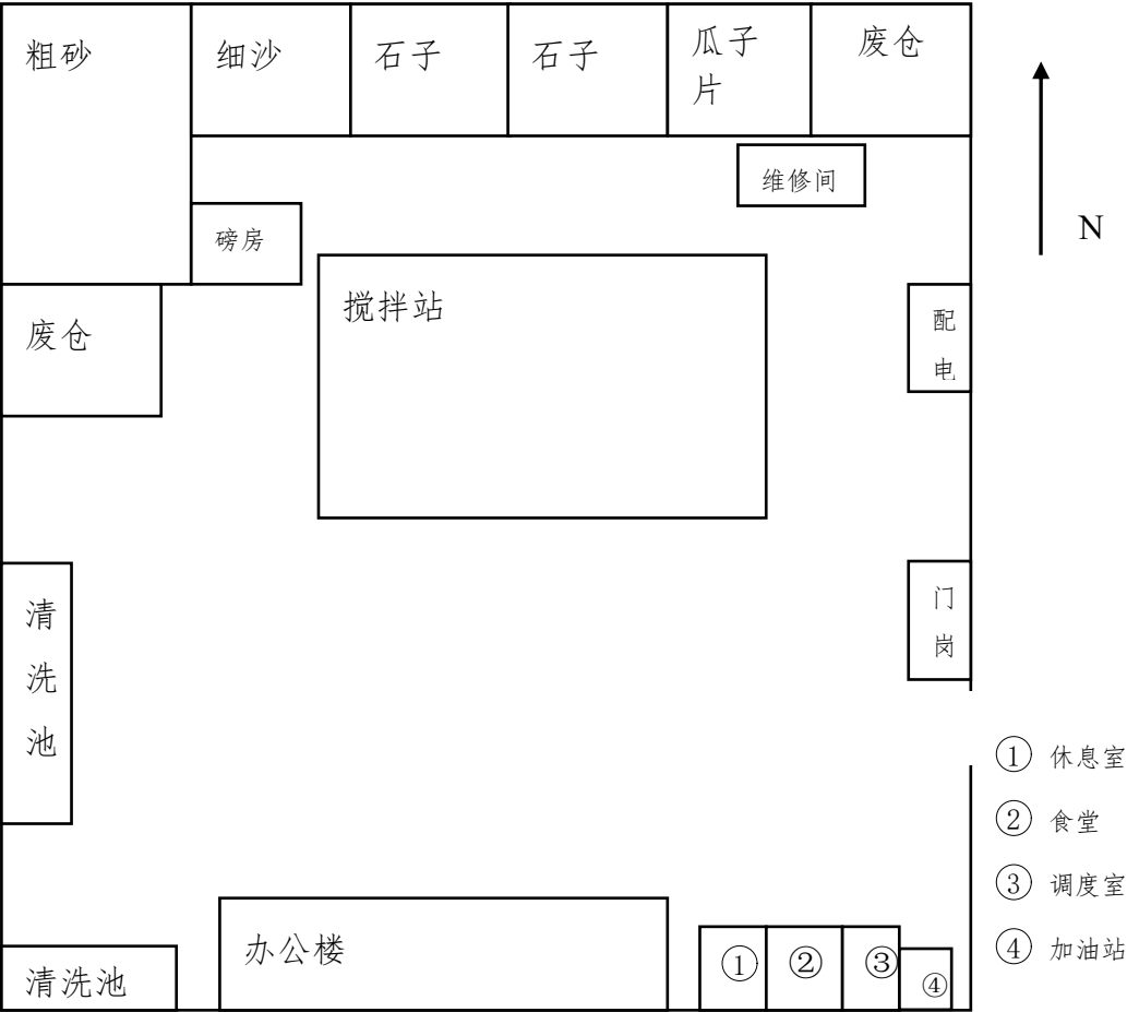
图 3-3 总平面布置图
