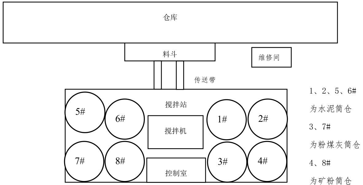
图 3-4 生产线设备布局图
