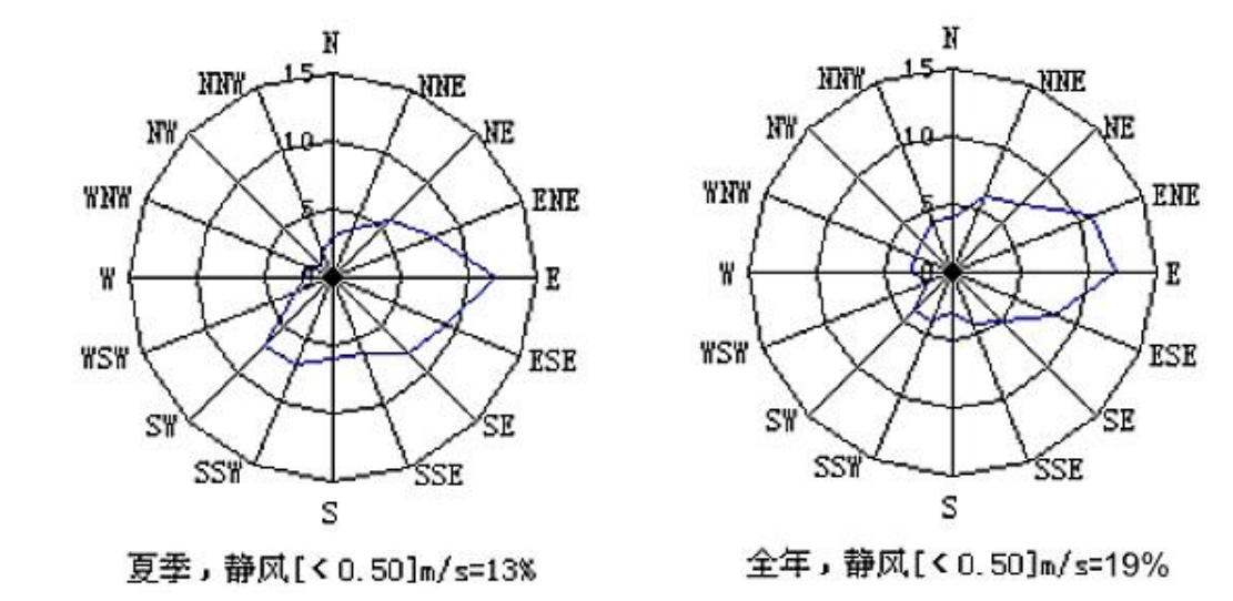
图 3-1 马鞍山市风向频率玫瑰图
